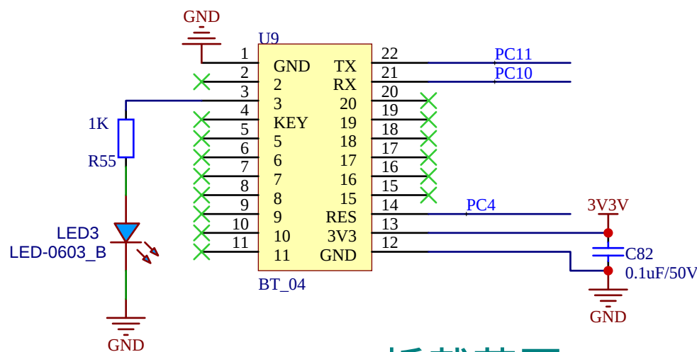
板载蓝牙
