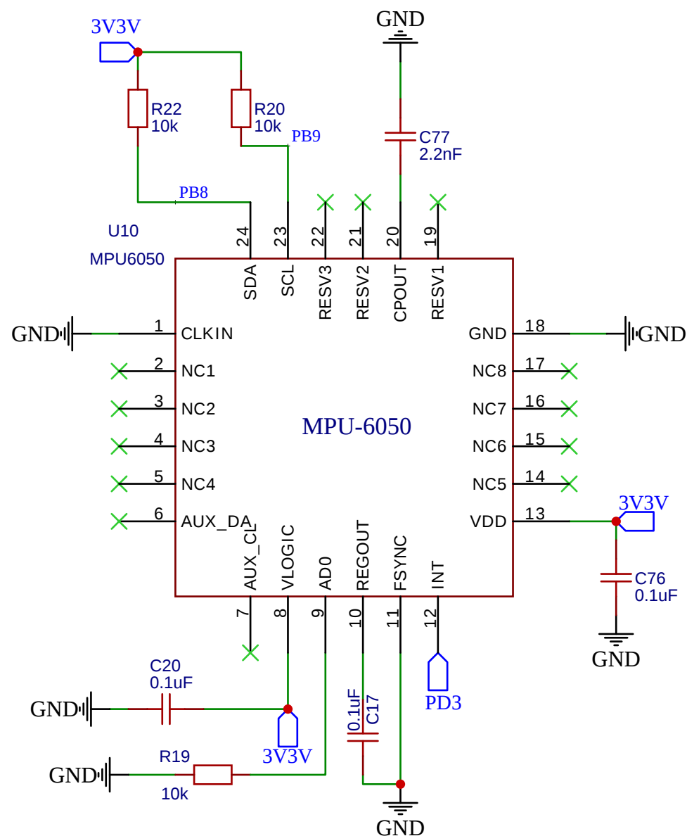
mpu6050电路
