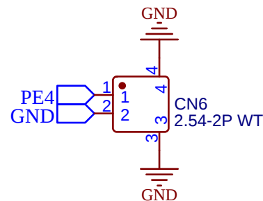
急停开关
