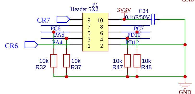
4路驱动接口
