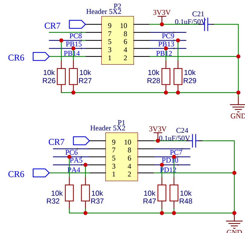
4路驱动接口
