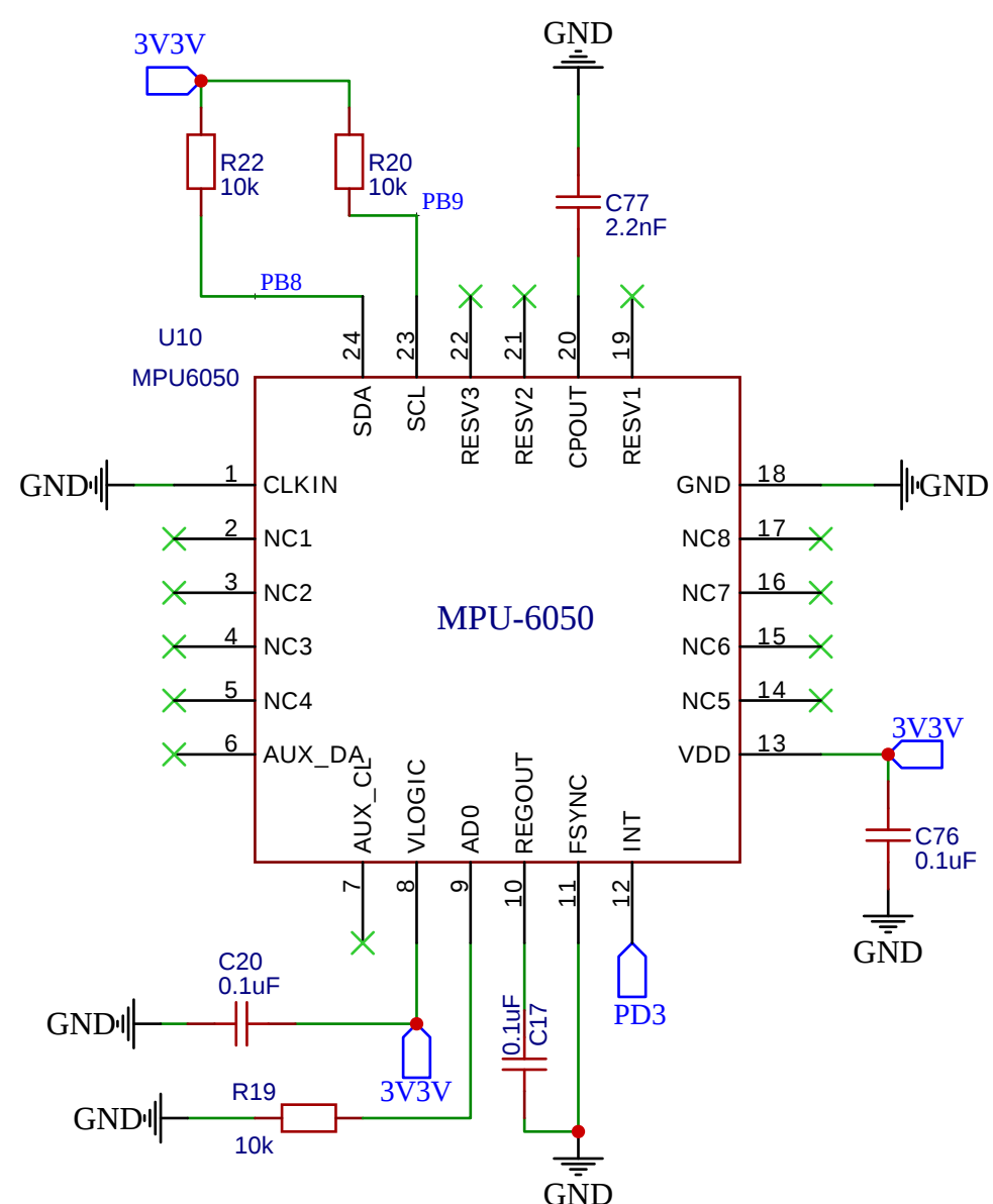
mpu6050电路
