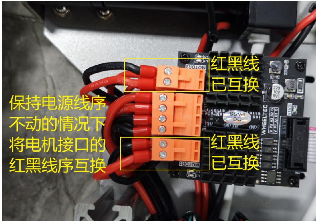
图 2-7 接线图
