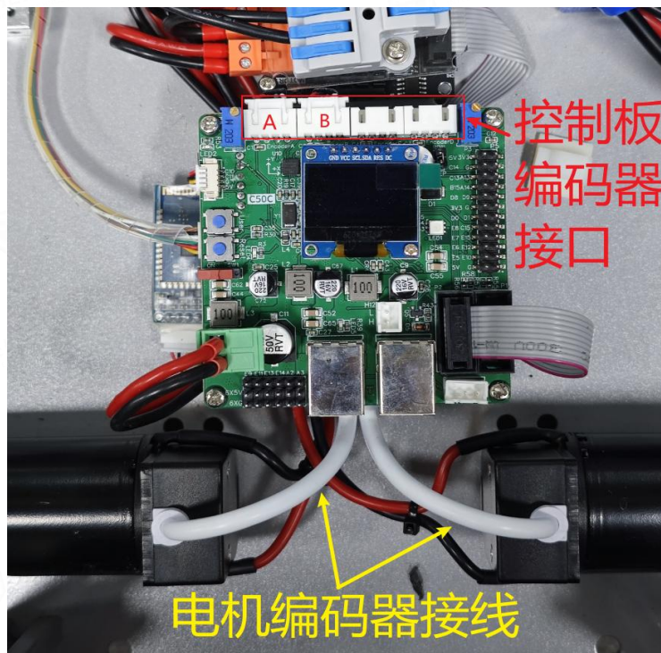
图 1-5 编码器接口及接线介绍
