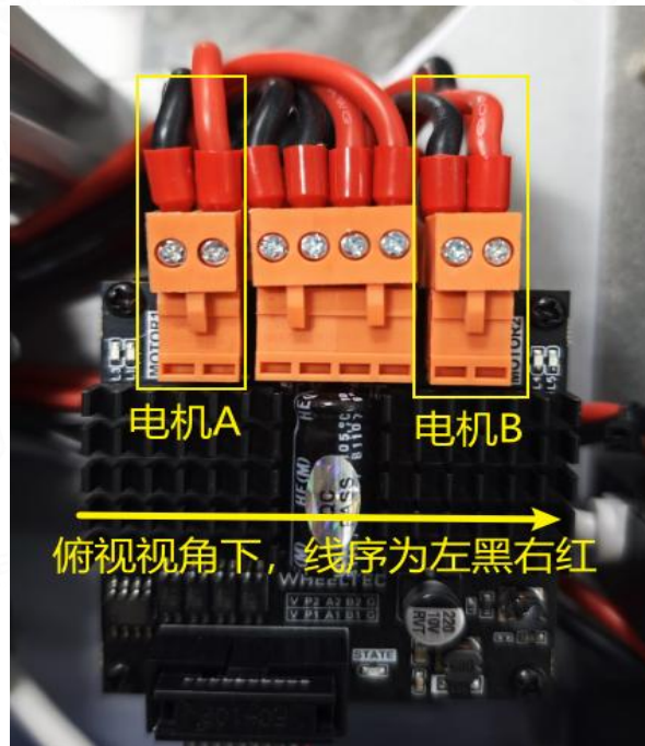
图 1-13 电机与电机驱动板接线图
