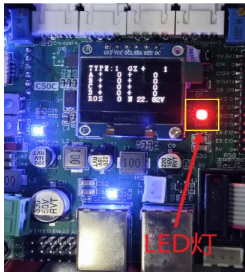
图 2-1 LED 灯位置
