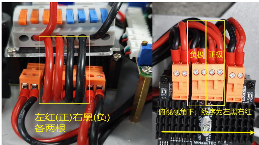
图 1-10 驱动板与集线器接线
