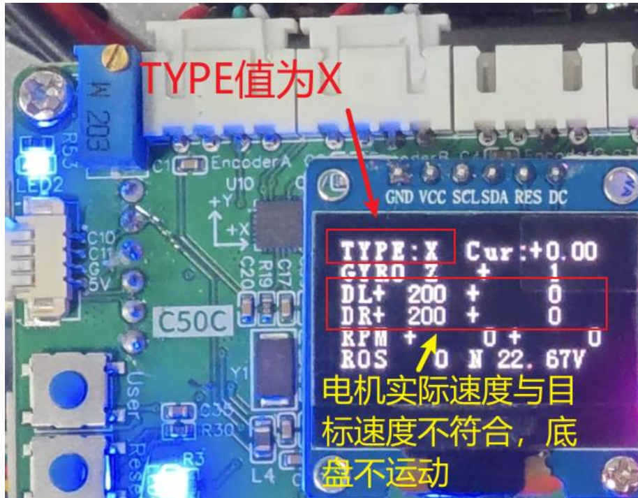
图 1-12 控制板与电机驱动板接口接反现象
