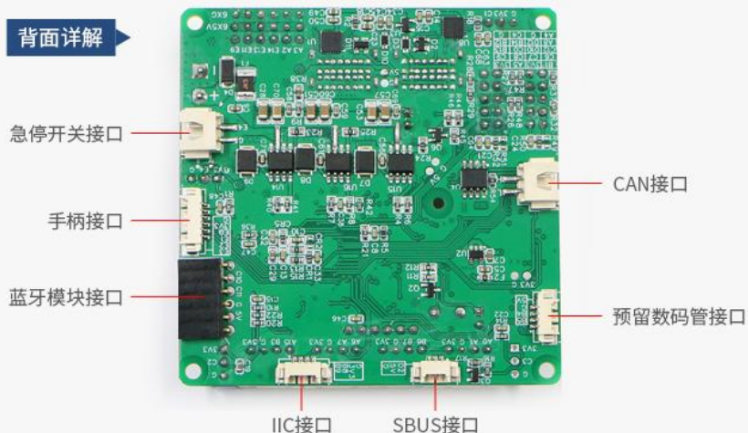
图 1-2 STM32 控制板详解
