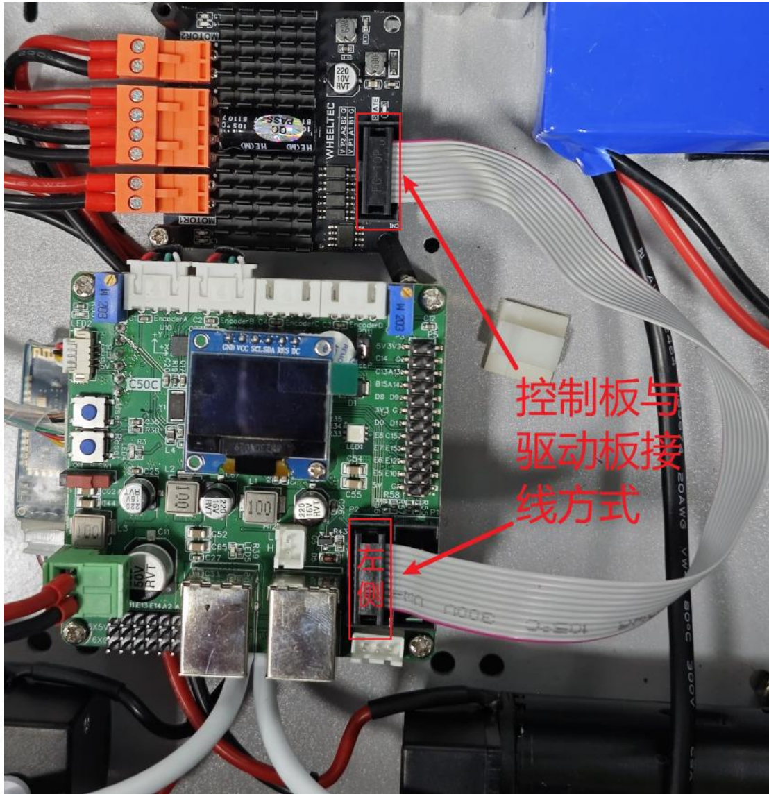
图 1-11 控制板与驱动板接线
