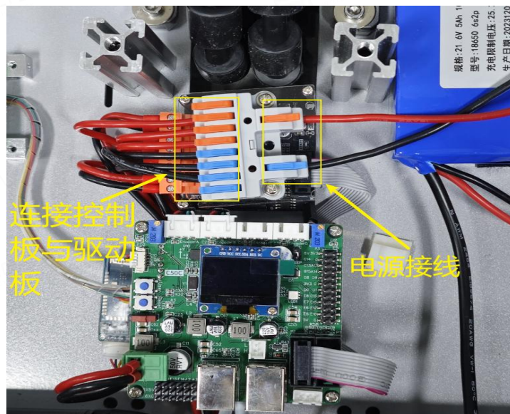
图 1-7 集线器
