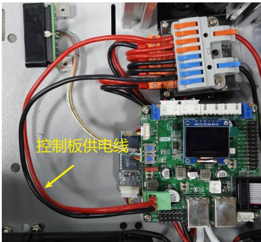
图 1-8 控制板与集线器接线
